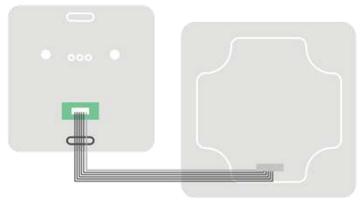
Ligação do teclado tátil com os módulos "W" (W-2ONOFF; W-1SHUTT; W-2VLESS; W-INPKEY).
